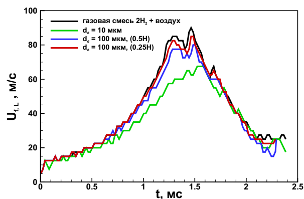
Рисунок 7. Хронограммы скорости ведущей точки фронта пламени U_{f,L} в канале шириной 20 мм, заполненном чистой стехиометрической смесью водород-воздух или газозвесью с содержанием капель воды диаметром 10 и 100 мкм и начальным расстоянием между каплями 1 мм. В скобках указана степень исходного заполнения канала каплями в поперечном направлении.
