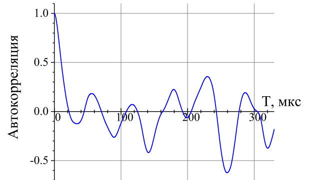
Рисунок 6. Автокорреляционная функция зависимости плавающего потенциала от времени.
