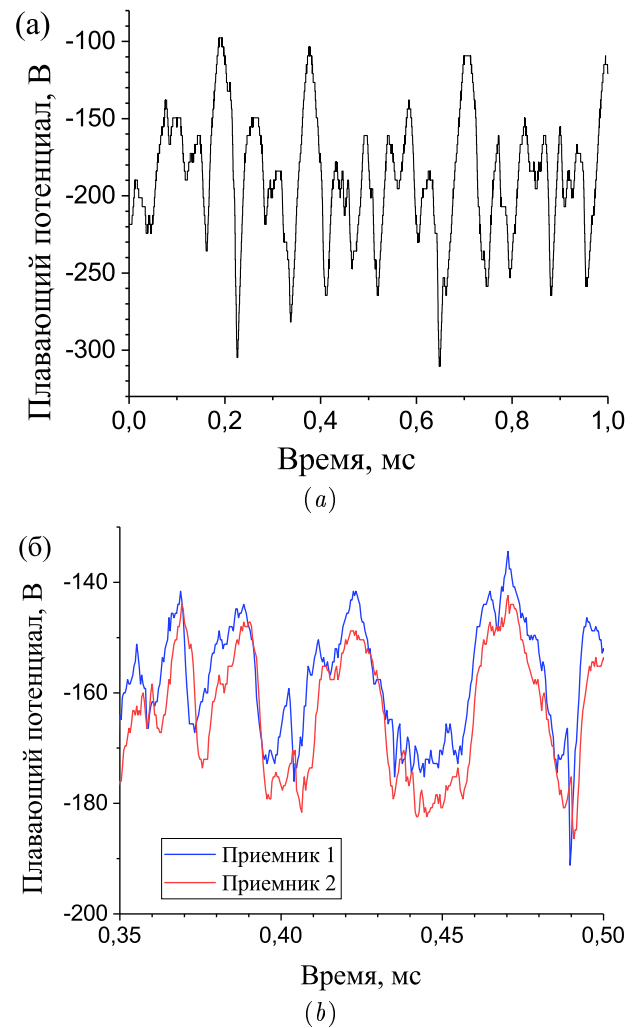
Рисунок 3. Характерный вид сигнала, полученного: (а) одиночным плавающим зондом, (б) регистрирующими элементами четырехканального зонда.
