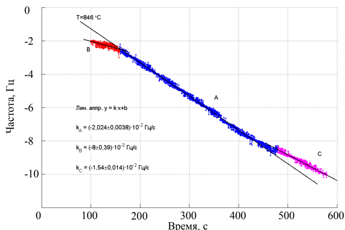
Рисунок 2. Изменение частоты кварцевого резонатора в процессе напыления свинца при температуре 846 °С в эффузионной ячейке. Участок кривой «А» соответствует открытой заслонке, а участки кривой «В» и «С» закрытой.
