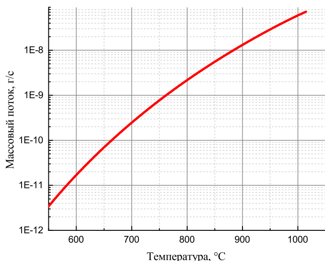
Рисунок 1. Зависимость массового потока, попадающего на площадку детектора, от температуры в эффузионной ячейке.
