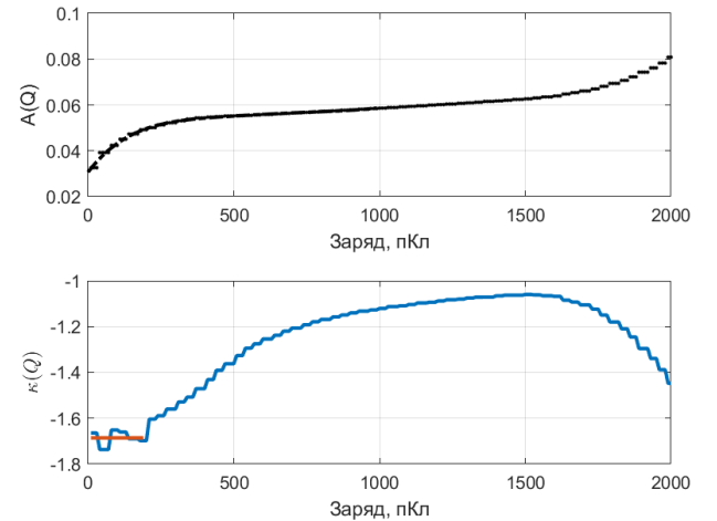
Рисунок 3. Зависимости A(Q) и \kappa(Q)
