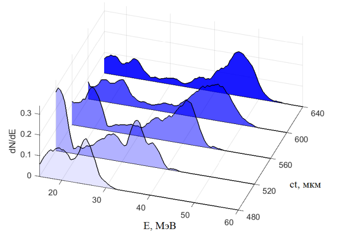
Рисунок 9. Зависимость распределения энергии электронов от времени для a_0 = 1 , n_0 = 0.04n_{cr} , x_M = 390 мкм.
