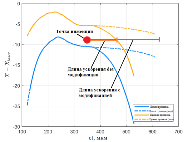
Рисунок 6. Эффект увеличения длины ускорения захваченных электронов путем модификации профиля плазмы за точкой инъекции ( a_0 = 1.6 , n_0 = 0.02n_{cr} ).
