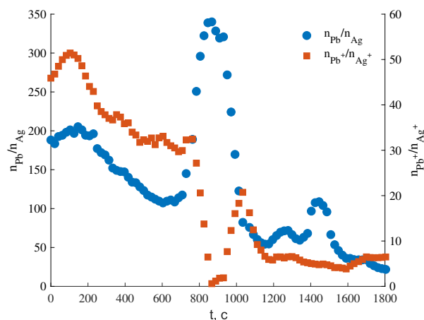
Рисунок 3. Поведение относительных концентраций атомов и ионов.
