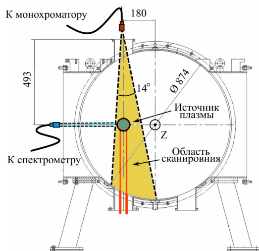
Рисунок 1. Схема эксперимента. Исследуемая плазменная струя источника (зеленый круг) параллельна оси Z . Регистрация излучения производится в плоскости, ей перпендикулярной.
