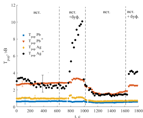
Рисунок 2. Поведение температур заселения Рб, Рб + , Ag, Ag + .
