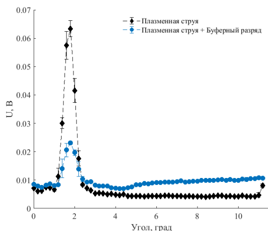
Рисунок 4. Профили излучения спектральной линии Рб II 537.2 нм.
