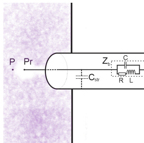
Рисунок 1. Схема измерительной части зонда.
