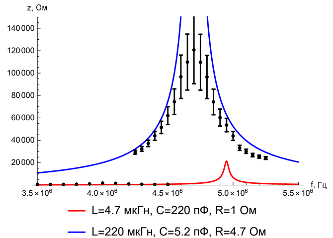
Рисунок 3. Импеданс катушки L = 220 мкГн с частотой собственного резонанса близкой к 5 МГц и контура, параметры которого выбирались, ориентируясь только на частоту генератора ( L = 4.7 мкГн, C = 220 пФ).
