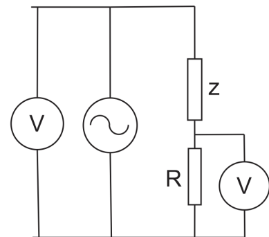
Рисунок 4. Схема измерений резонансной частоты колебательного контура.
