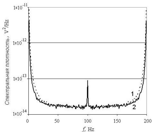
Рисунок 2. Фурье-спектры шума, показывающие влияние демпфирования (ослабление/устранение микросейсма).
