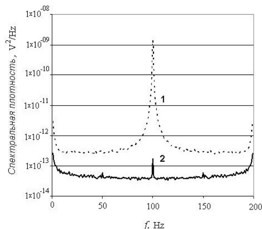
Рисунок 3. Фурье-спектры шума, показывающие влияние экранирования.
