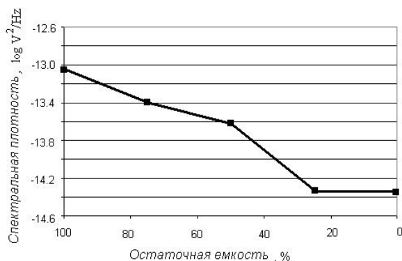
Рисунок 5. Зависимость усредненной спектральной плотности шума от остаточной емкости ЛХИТ.
