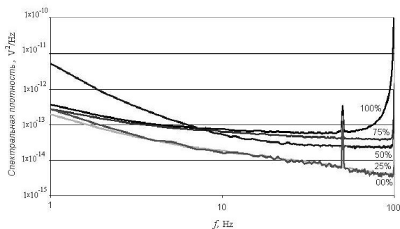
Рисунок 4. Усредненные размерные спектры шума для разных степеней разряженности ЛХИТ.
