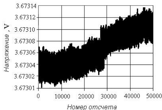
Рисунок 1. Измерения шумовых характеристик ХИТ при воздействии на них термоизлучающего устройства.
