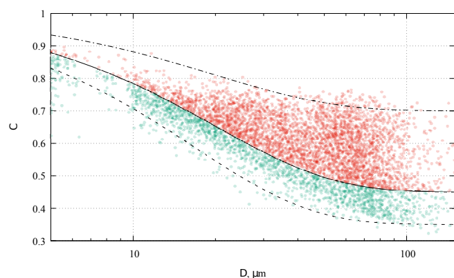
Рисунок 3. Распределение отношения интенсивностей C_1(D) (---), C_2(D) (— · —) Сплошной линией показана выбранная граница отсева изображений каплей C(D) .
