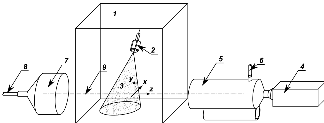
Рисунок 1. Схема экспериментальной установки. 1 — прозрачная емкость, 2 — форсунка, 3 — факел распыла жидкости, 4 — видеокамера, 5 — микроскоп, 6 — видеоискатель, 7 — оптический преобразователь, 8 — оптический волновод, 9 — оптическая ось.
