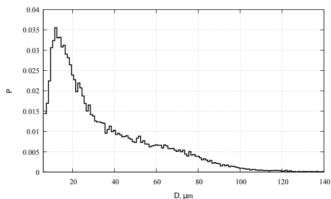
Рисунок 4. Пример построенной вероятности P(D) при p_w = 6 бар.
