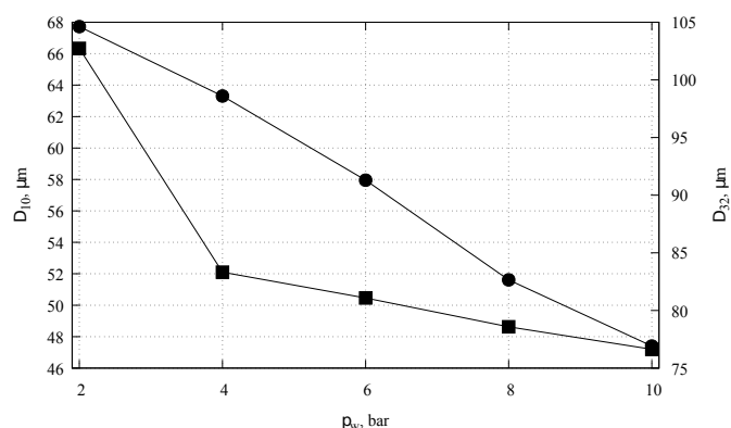
Рисунок 5. Зависимость параметров D_{10} (■) и D_{32} (●) от давления воды p_w .
