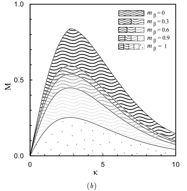
Рисунок 1. Область устойчивого существования цепочечной конфигурации двух пылевых частиц, взаимодействующих с потенциалом (2), в зависимости от значения числа Маха M и параметра экранирования \kappa : (a) m_\beta = 0 , штриховая, сплошная и пунктирная кривые соответствуют соотношениям (12), (11) и (10); (b) область значений, удовлетворяющих условиям (10)–(12), с ростом относительной величины градиента радиального электрического поля m_\beta от 0 до 1.
