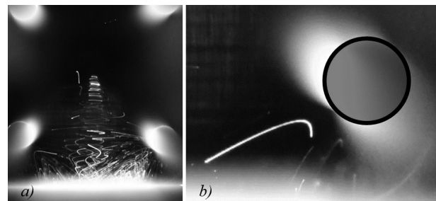
Рисунок 5. Траектория частиц в электродинамической ловушке (вид с торца) при следующих значениях напряжения: (a) U_a = 4 кВ; (b) U_a = 3 кВ.
