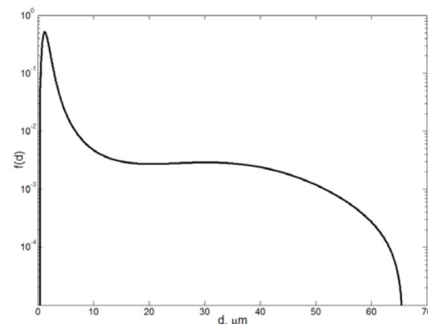
Рисунок 2. Распределение частиц по размерам \text{Al}_2\text{O}_3 .
