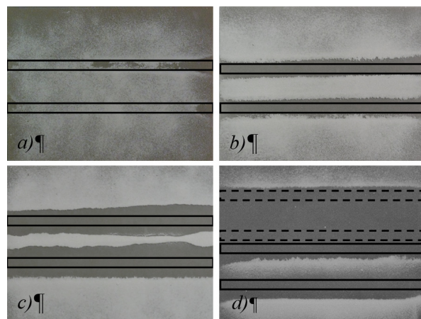
Рисунок 4. Фотографии стеклянной подложки с частицами \text{Al}_2\text{O}_3 , помещенной на различных расстояниях l от электродов ловушки при U_a = 5 кВ: (a) l = 1 см, (b) и (d) l = 0.5 см, (c) l = 0.15 см. Проекция электродов обозначены сплошными линиями. На изображении (d) начальная проекция электродов ловушки на подложку обозначена штриховыми линиями, конечная — сплошными.
