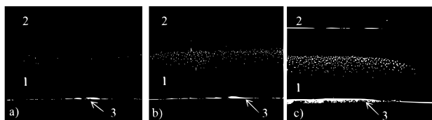
Рисунок 3. Захват частиц \text{Al}_2\text{O}_3 со стеклянной подложки, расположенной на расстоянии 0.5 см от электродов ловушки: (a) U_a = 3.5 кВ, (b) и (c) U_a = 5 кВ; 1, 2 — электроды ловушки, 3 — стеклянная подложка с частицами; (a) и (b) — изображения центральной части ловушки, (c) — изображение у открытого торца ловушки.
