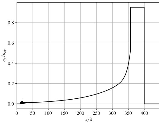
Рисунок 7. Пространственное распределение начальной концентрации электронов по оси OX при фокусировке лазерного импульса на расстоянии 172.5 мкм от начала мишени.
