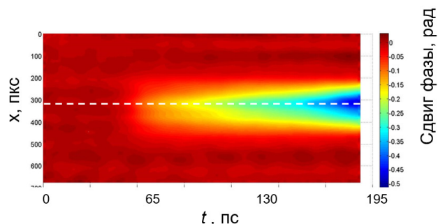
Рисунок 1. Пространственно-временное распределение фазы диагностического импульса. Энергия нагревающего лазерного импульса E = 13 мкДж, длительность 0.8 пс. Пространственный масштаб в плоскости мишени по вертикальной оси равен 0.3 мкм/пкс. Цветовая шкала дана в радианах.
