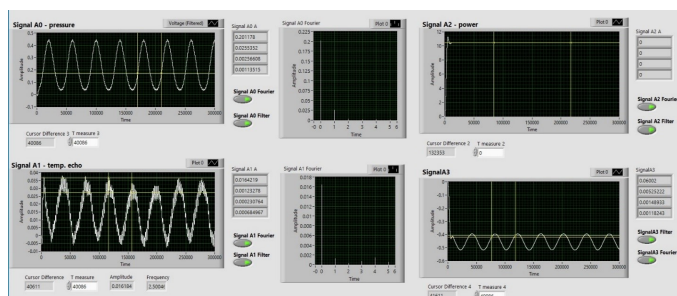
Рисунок 3. Компенсация с удвоенным температурным откликом. Колебания давления и мощности электрического тока имеют одинаковую фазу.
