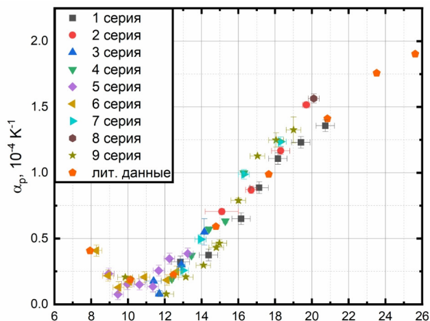
Рисунок 5. Температурная зависимость КТР в абсолютных величинах.
