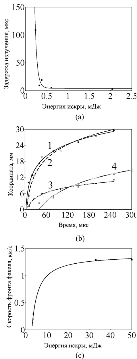
Рисунок 4. Экспериментальные результаты: (a) — аппроксимация задержки оптического проявления горения из области реакции от энергии электроискрового инициирования; (b) — x - t диаграммы фронтальной области свечения для разных значений энергии искрового инициирования смеси с наноразмерными компонентами (линия 1 — 50 мДж, линия 2 — 33 мДж, линия 3 — 3.6 мДж и с микроразмерными компонентами, линия 4 — 3.3 мДж); (c) — аппроксимация начальной скорости формирования факела от энергии искрового инициирования (■ — результаты для смеси наноразмерными компонентами, □ — результаты для смеси микроразмерными компонентами).
