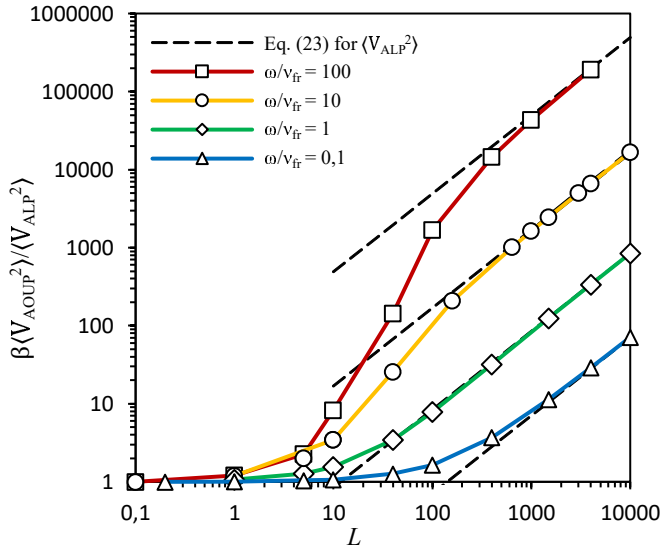
Рисунок 2. Зависимость отношения \beta \langle V_{\text{AOUP}}^2 \rangle / \langle V_{\text{ALP}}^2 \rangle от L = \omega_0 / \omega \nu_{\text{fr}} при различных \omega / \nu_{\text{fr}} . Символы — \beta \langle V_{\text{AOUP}}^2 \rangle / \langle V_{\text{ALP}}^2 \rangle_{\text{sim}} , где значения \langle V_{\text{ALP}}^2 \rangle_{\text{sim}} измерены в результате численного моделирования динамики активной частицы с использованием уравнений (1), (4) и (5). Штриховые линии — аппроксимация (23) для \langle V_{\text{ALP}}^2 \rangle .
