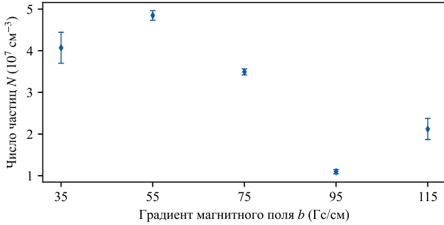
Рисунок 7. Зависимость числа частиц в облаке нейтральных атомов от градиента магнитного поля в центре МОЛ.
